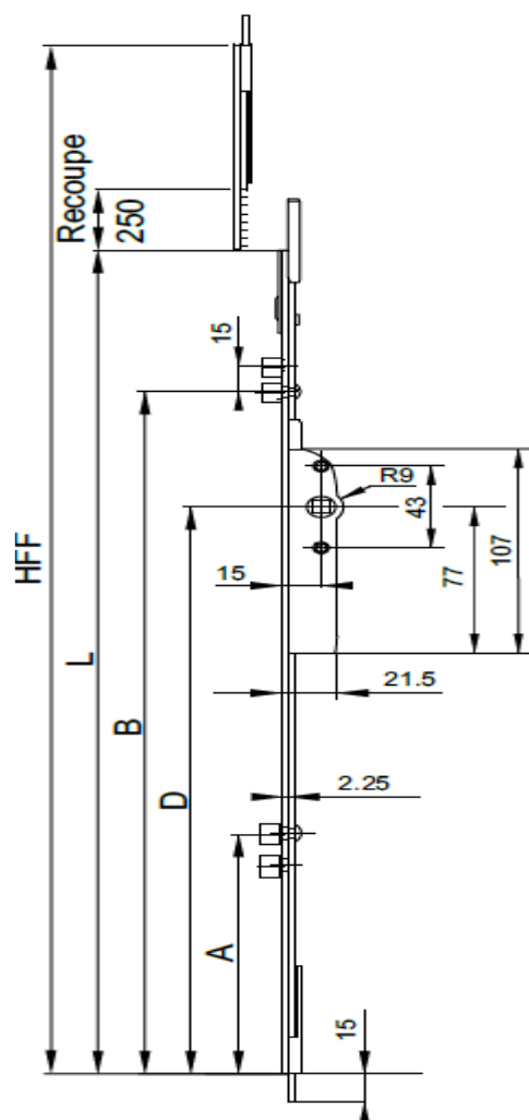
Crémone F15 ajustable à galet G-20466-**-0-1
