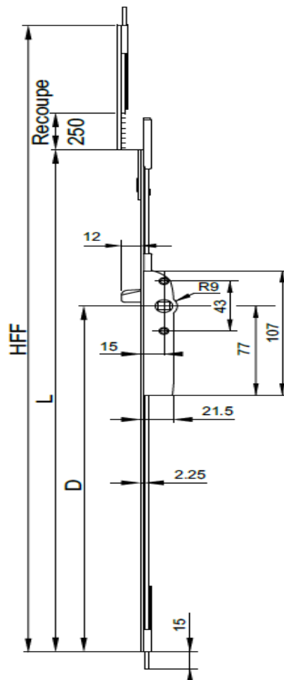
Crémone F15 ajustable à panneton G-20395-**-0-1
